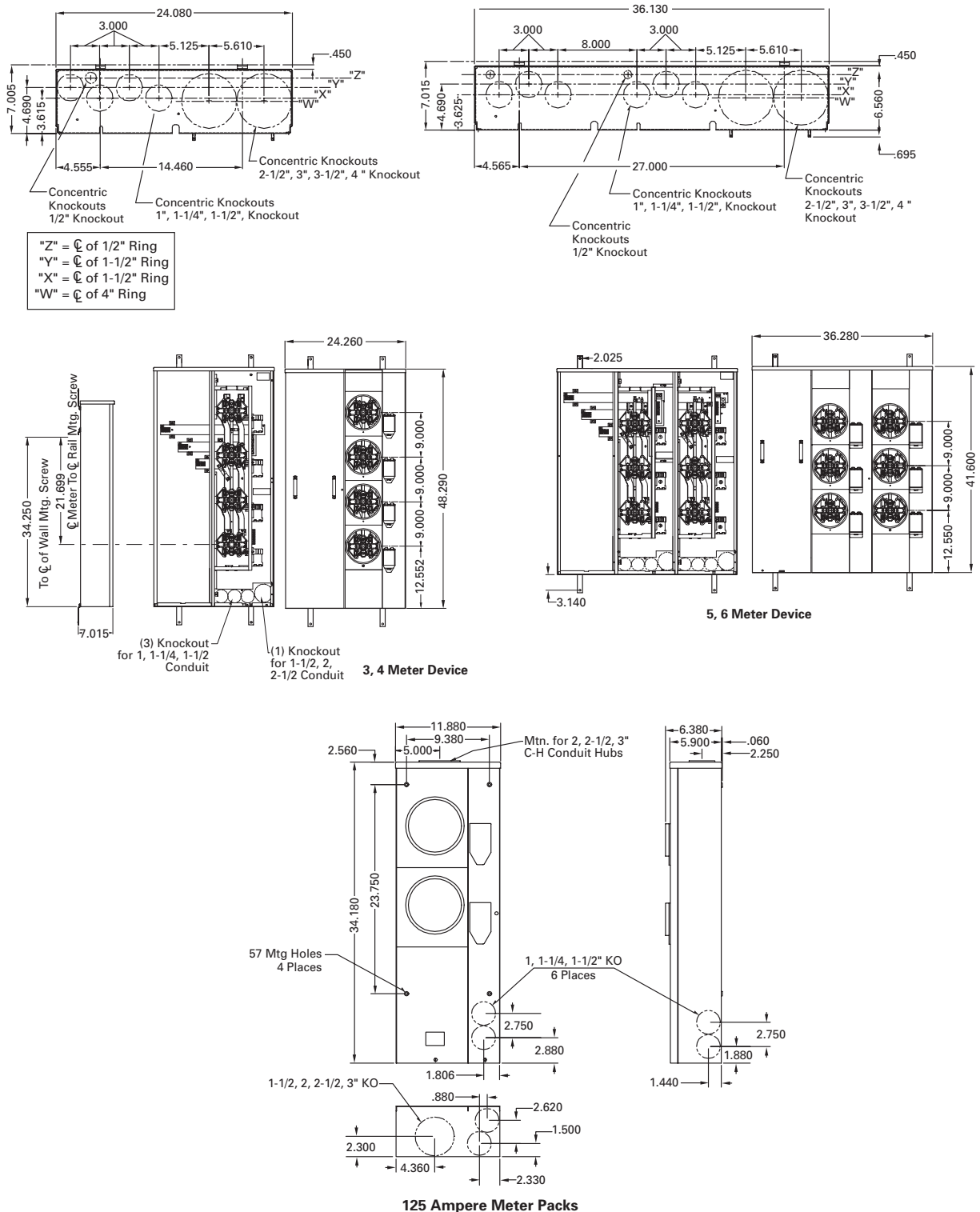
Figure 2. 125 Ampere Maximum Tenant Breaker
